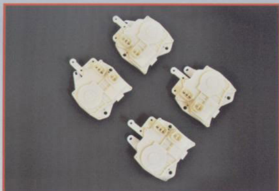
ACCORD 98(2.0/2.3) 廣本 2.3/CG5 ACTUATOR ASSY., DOOR LOCK SK3516-ACD98 72115-S84-A013 (FR) SK3517-ACD98 72155-S84-A013 (FL) SK3518-ACD98 72615-S84-A013 (RL) SK3519-ACD98 72655-S84-13 (RR)
