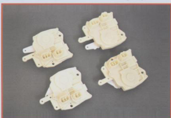
ACCORD 98(3.0/V6) 廣本 3.0/CG1 SK3516-ACD98-A 72115-S84-A11 (FR) SK3517-ACD98-A 72155-S84-A11 (FL) SK3518-ACD98-A 72615-S84-A11 (RR) SK3519-ACD98-A 72655-S84-A11 (RL)
