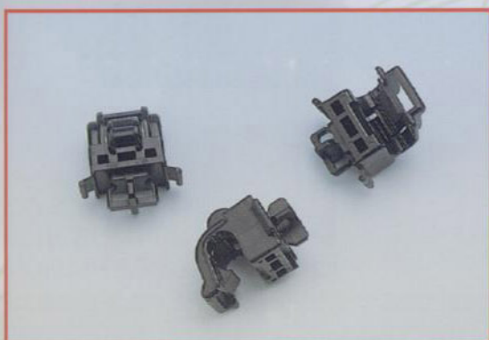
ACCORD 90 引擎蓋支撐桿固定座 HOLDER ROD. HOOD STAY SK6260-ACD90 90677-SE0-003
