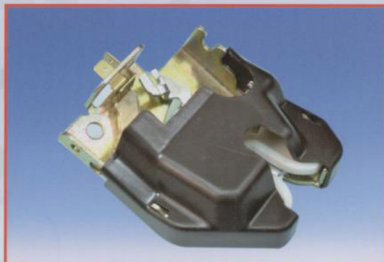
FIT 05 4 DOOR 廣本 三廂 GD6 後箱蓋六角鎖 LOCK, TRUNK SK6235-HFIT054D 74801-SAA-E21
